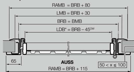
Coupe horizontale
